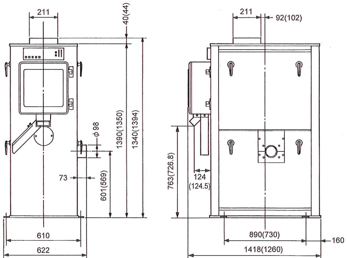
図 7-1 寸法図
